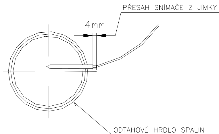
UMÍSTĚNÍ SNÍMAČE TEPLoty SPALIN V JÍMCE ODTAHOVÉHO HRDLA POHLED ZE ZADU
